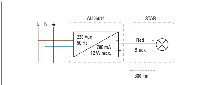
ALI05014 : Wiring diagram Schéma de câblage
