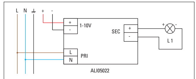
ALI05022 : Wiring diagram Schéma de câblage
